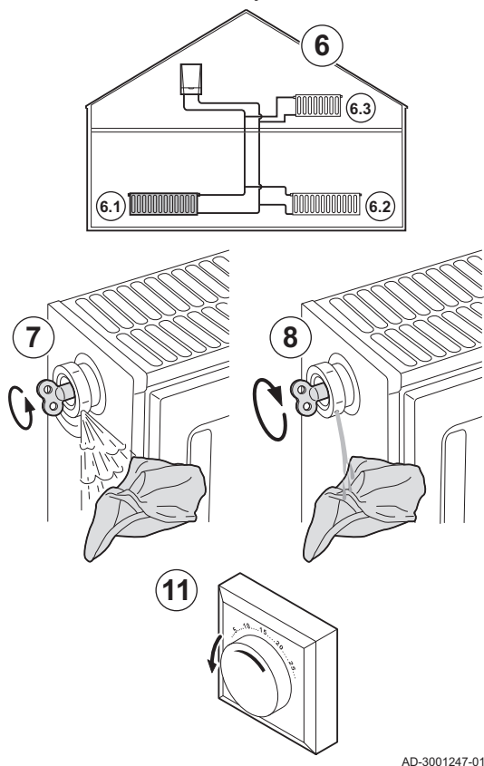
Рис.14 Удаление воздуха из системы
