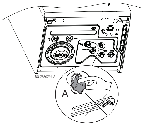
Рис. 67 Заполнение установки
