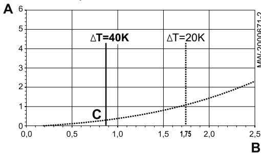
Рис.2 Потери давления для C140 – 45
