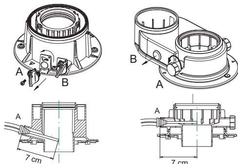
Рис. 177 Тип фитингов – измерительный отвод дымовых газов
