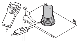
Рис. 178 Примеры проверок сгорания
