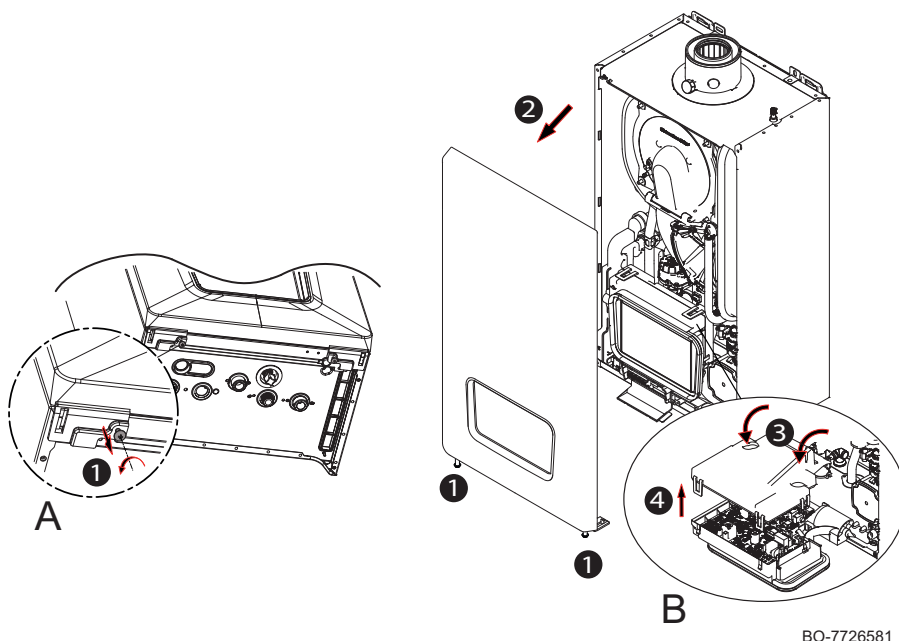
Рис. 161 Доступ к электрическим соединениям
