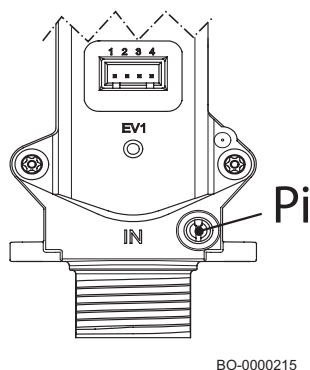
Рис. 176 Газовый клапан
