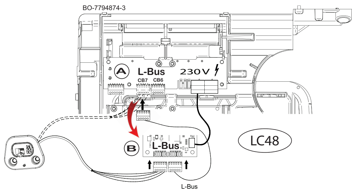
Рис. 166 Подключение платы дополнительного оборудования в котле
