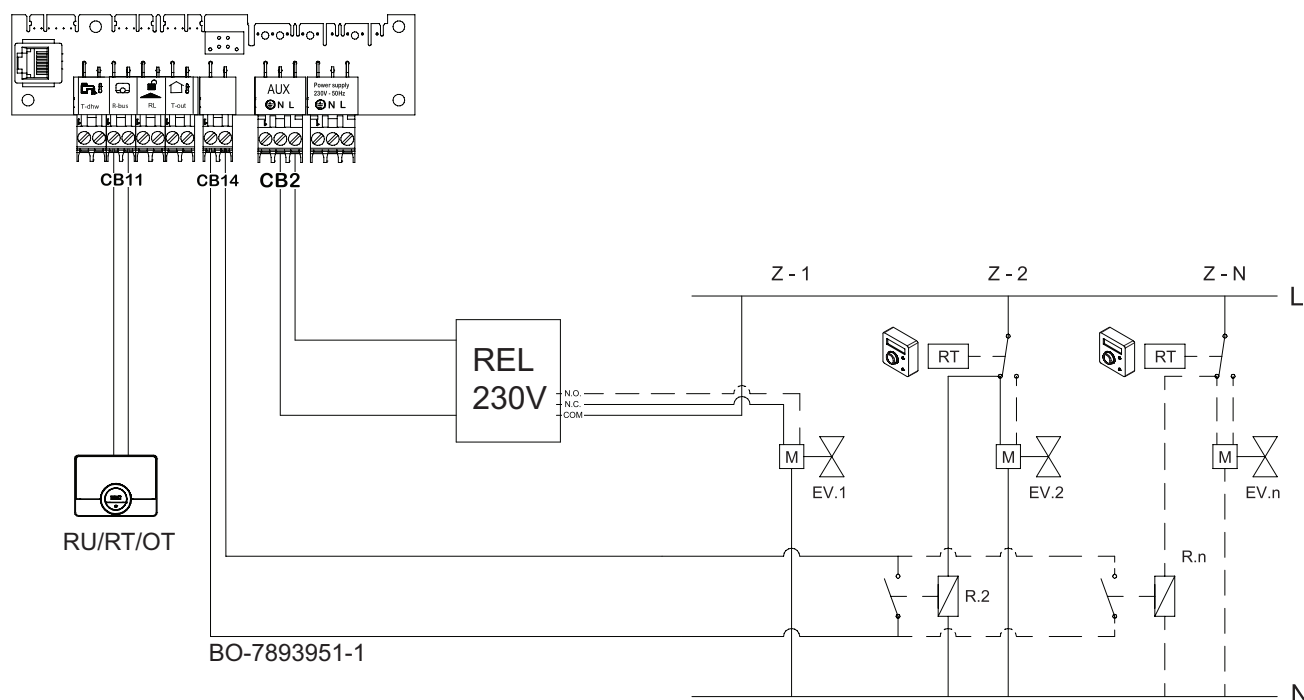
Таб 155 Описание входов/выходов
