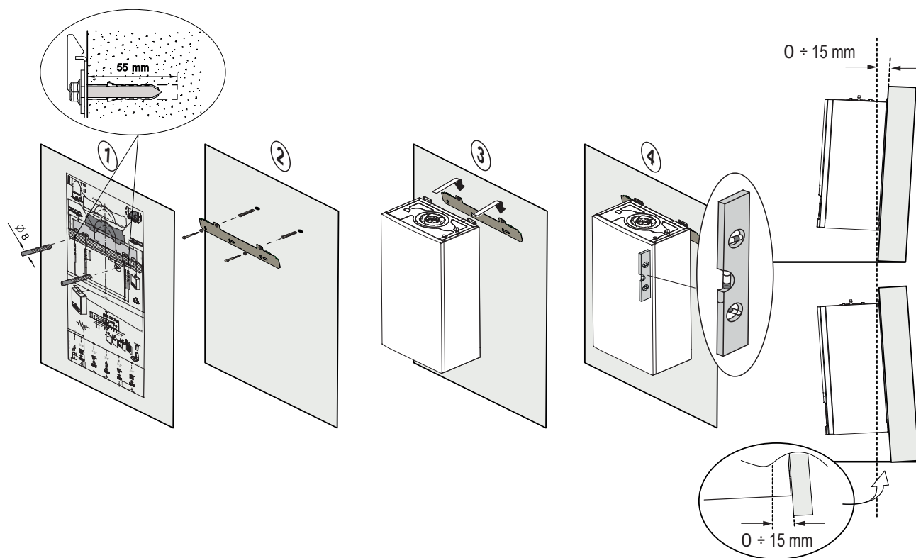
Рис. 148 Установка на стене
