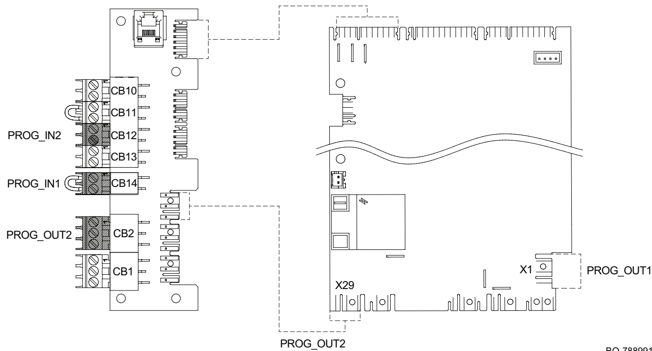
Рис. 167 Схема конфигурации программируемого выхода/входа
