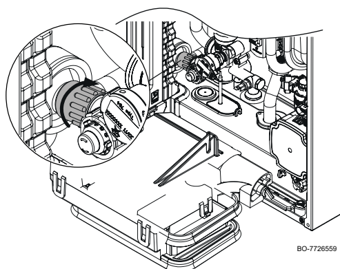
Рис. 174 Слив установки
