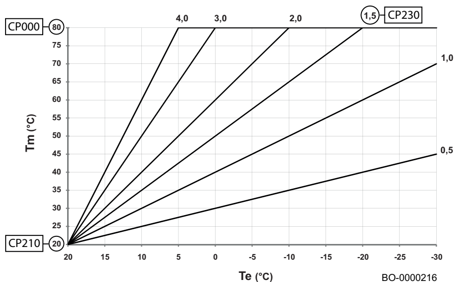
Рис. 191 Отопительный график
