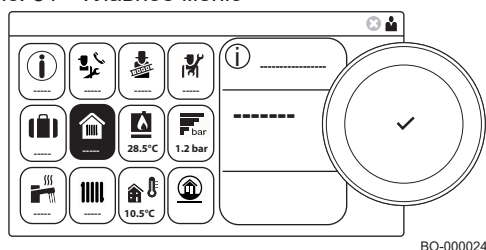
Рис. 31 Главное меню
