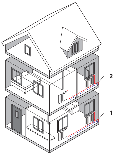
Рис. 36 Две зоны
