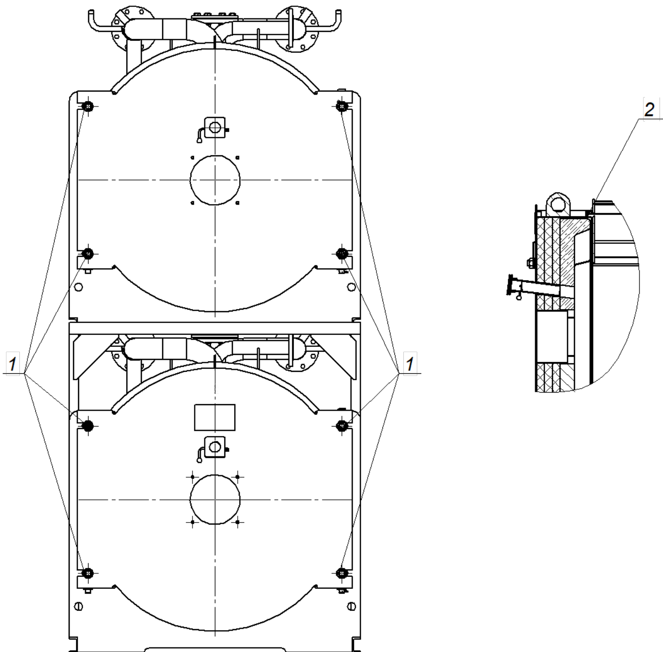
Рисунок 10. Передние крышки.
